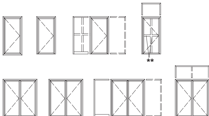
Rahmenbauweise
