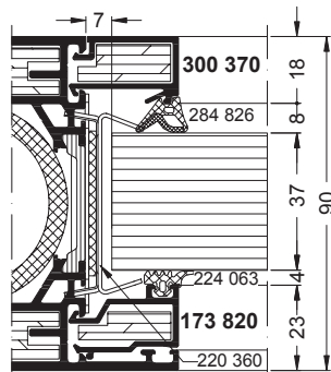
SchücoFlam 90 C
