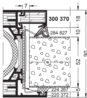
Stahlblech-Panel
