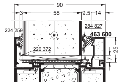
Glas / Alu-Paneel
