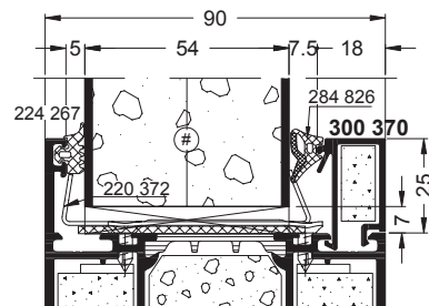
Alu-Paneel
