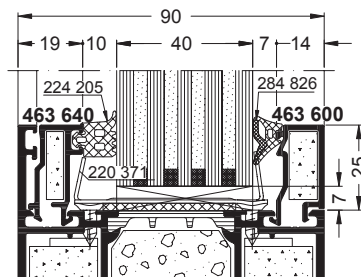
SchücoFlam 90 C
