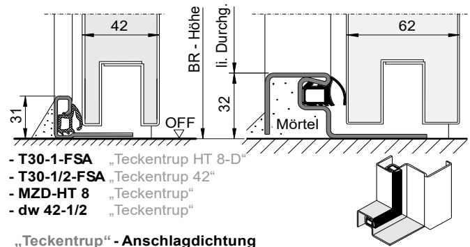
„Teckentrap“ - Anschlagdichtung (nicht zugelassen für Flucht- und Rettungswege)
