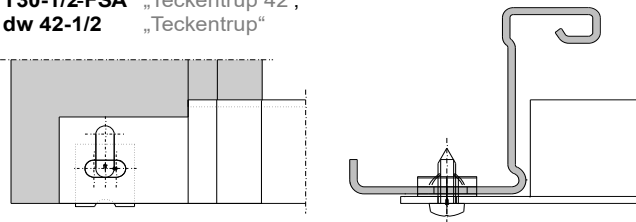
Bodenanschluss mit 4-seitiger Zarge und 4-seitiger Falz bei Klappen und Türen
